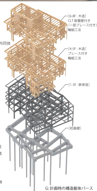
G: 計画時の構造躯体パース
